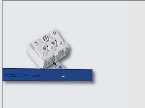
2. Montageschritt
