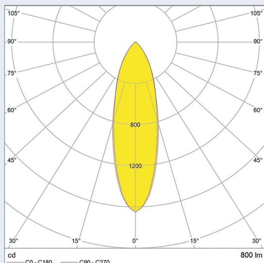
Lichtverteilung mit Philips Fortimo LED Strip OC
